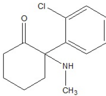
Ketamine
